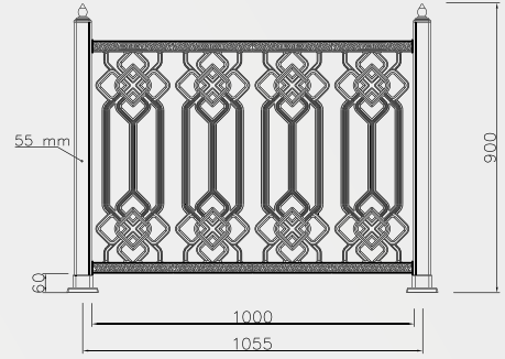
Alüminyum Ayak Aluminum Foot
