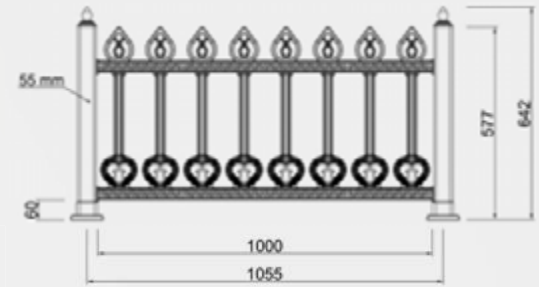
Alüminyum Ayak Aluminum Foot
