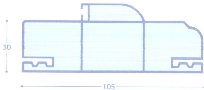
N/2 - PROFIL CADRE 105MM
