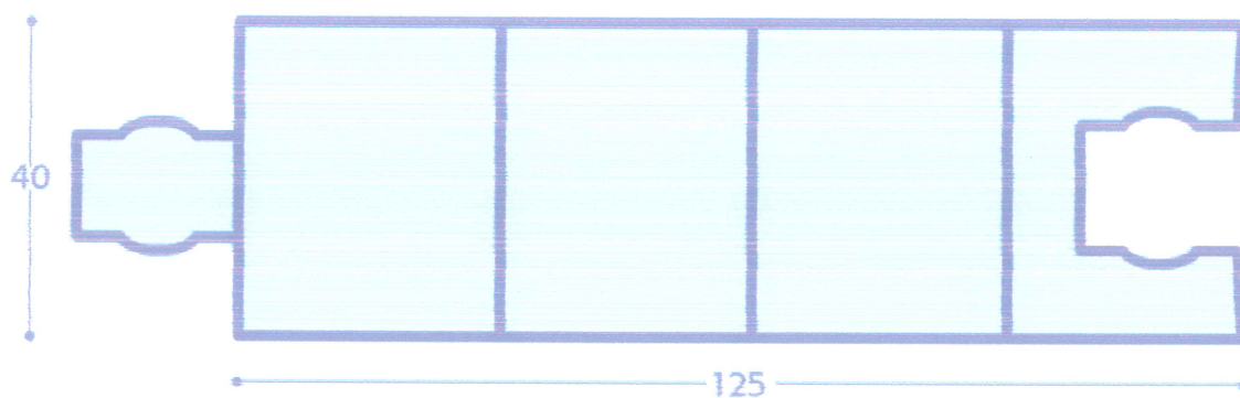
A/1 - PANNEAU DE PORTE DE 125X40MM
