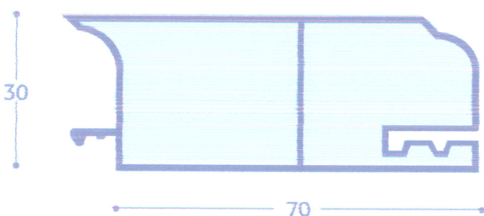
N/3 - ELARGISSEMENT PROFIL DE CADRE 70MM
