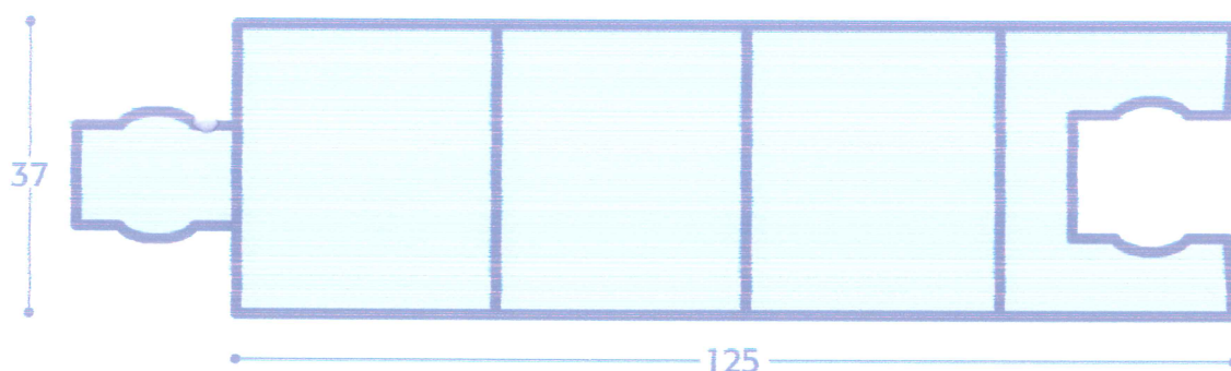
A/37 - PANNEAU DE PORTE DE 125X37MM PVC recyclé
