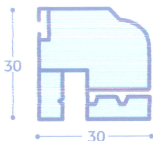
N/18 - PROFIL CADRE "SCRIGNO"
