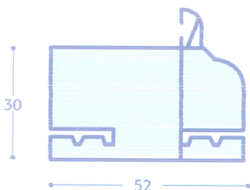
N/13 - PROFIL CADRE 52MM
